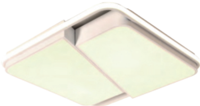
Plafon Yone Wh Plafon Branco em LED TEMPERATURA DA COR 3000K POTÊNCIA 72W DIMENSÕES 51cm x 51 cm x 06cm
