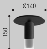
PLAFON COD.: LS5P
