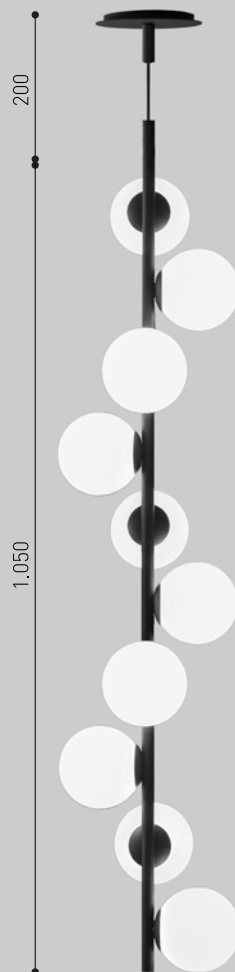
PENDENTE FLEXÍVEL COD.: CENT2PF
