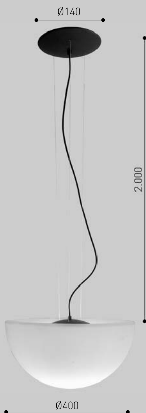
1/2 ESFERA Ø 400mm COD.: P035P
