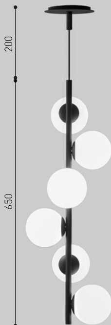
PENDENTE FLEXÍVEL COD.: CENT8PF
