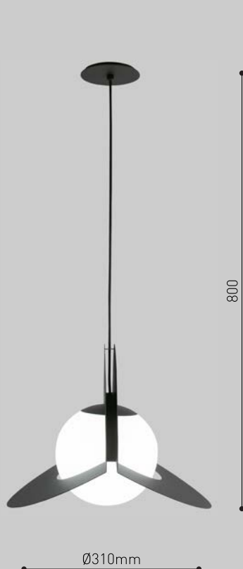
PENDENTE - ESFERA Ø160 COD.: BAU1P
